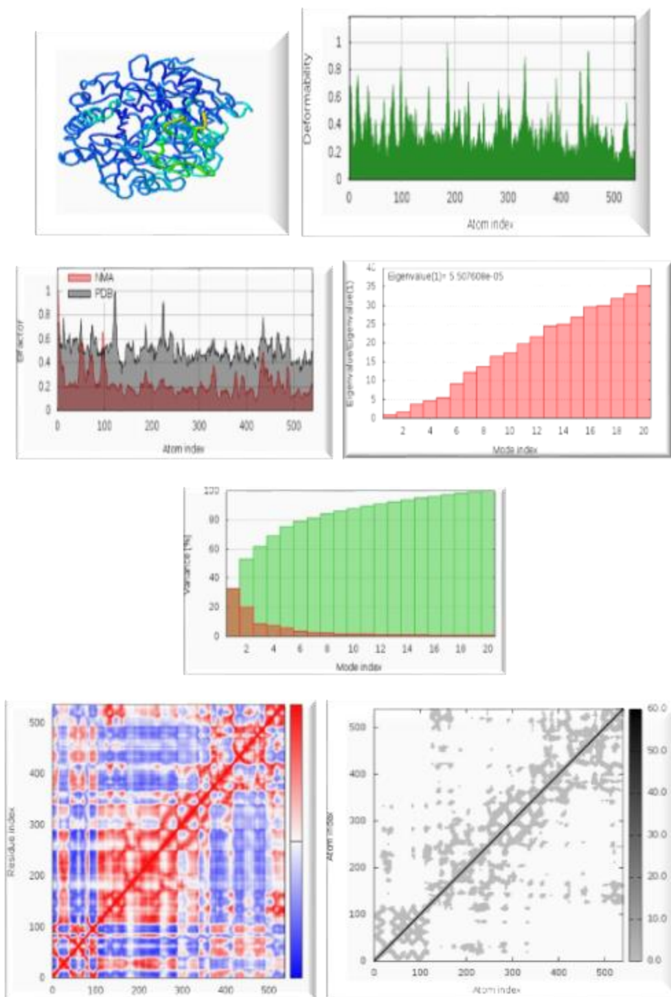
Figure 49 : Résultats de la simulation de la dynamique moléculaire du récepteur BETATHUJONE-5GQB
