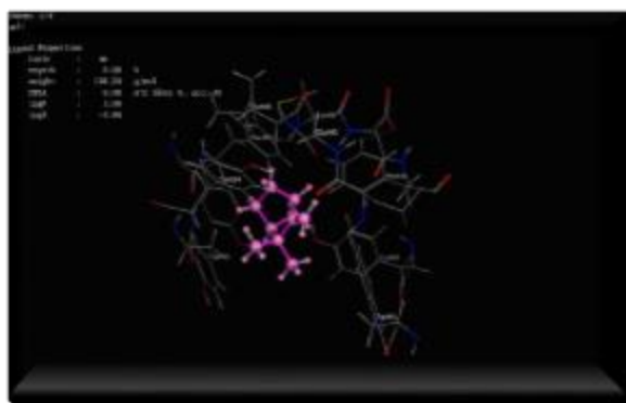
Complexe 5YDJ- Camphène.
