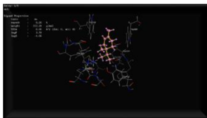
Complexe 5GQB-Terpinène-4-Ol.
