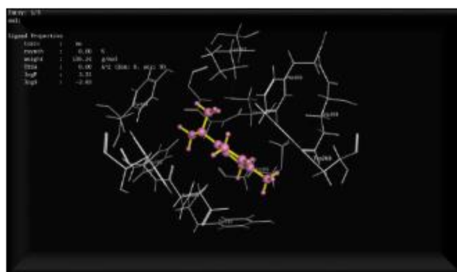
Complexe 5GQB-Gamma-Terpinène.
