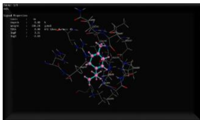
Complexe 6B04-Gamma-Terpinène.
