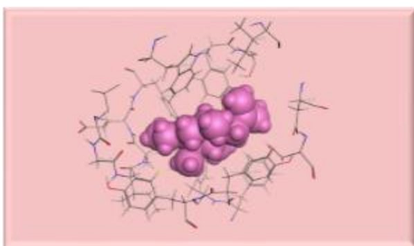
Complexe 5YDJ-Ligand de Co-cristallisation N-Acétyleglucosamine
