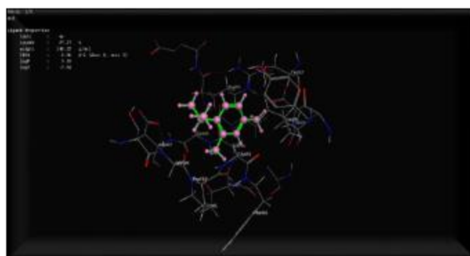
: Complexe 4ARX-Thymol.
